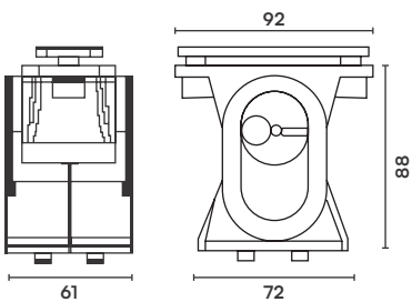
Steun
