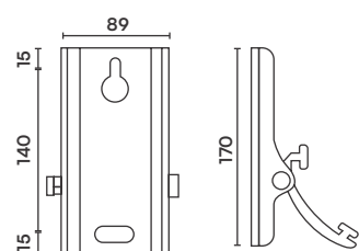
Muursteun
