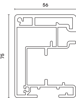
Geleider
