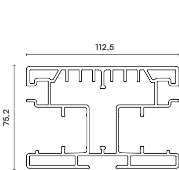
Koppelgeleider
