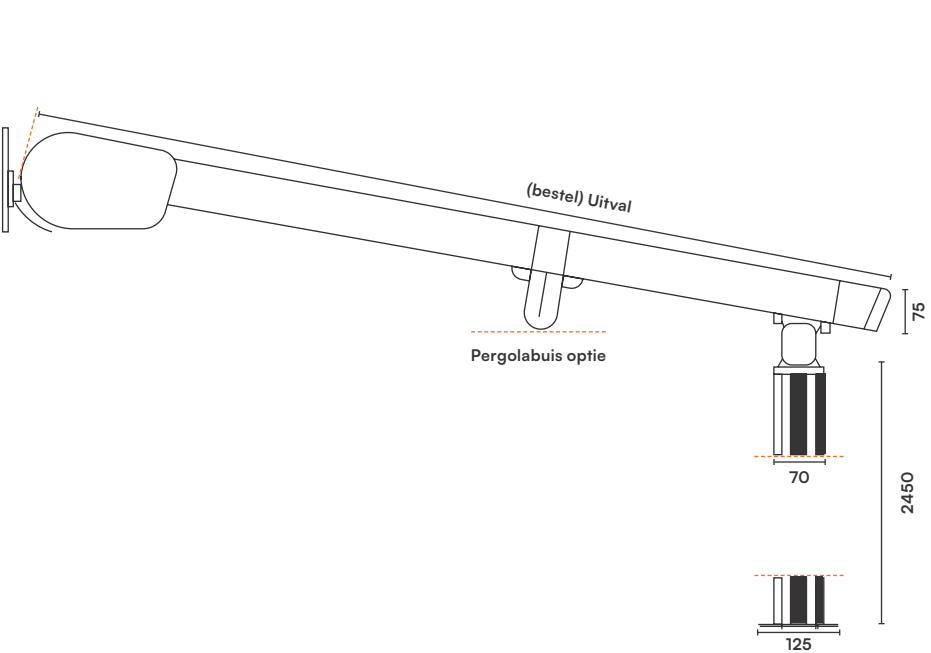
Pergola
